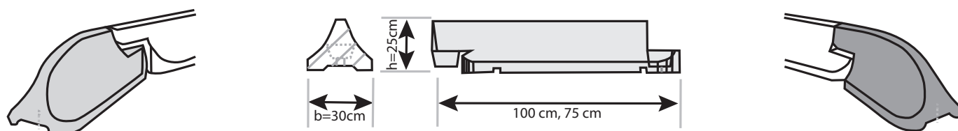
Elementi per isole spartitraffico - altezza 25 cm
