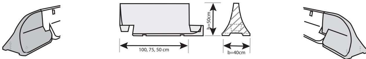
Elementi per isole spartitraffico - altezza 50 cm
